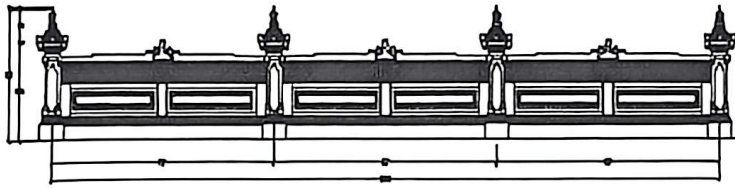
TAMPAK DEPAN PAGAR
