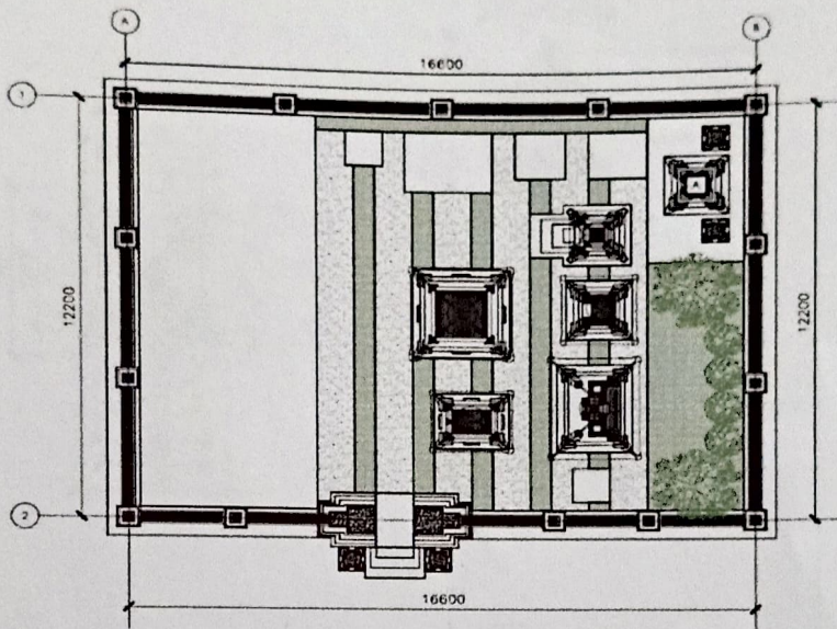
GAMBAR PERENCANAAN
