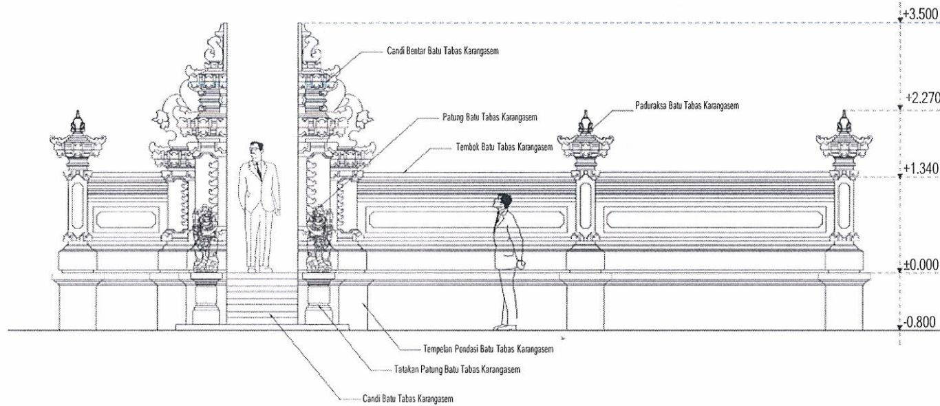
RENCANA CANDI BENTAR & TEMBOK PENYENGKER Skala 1 : 50
